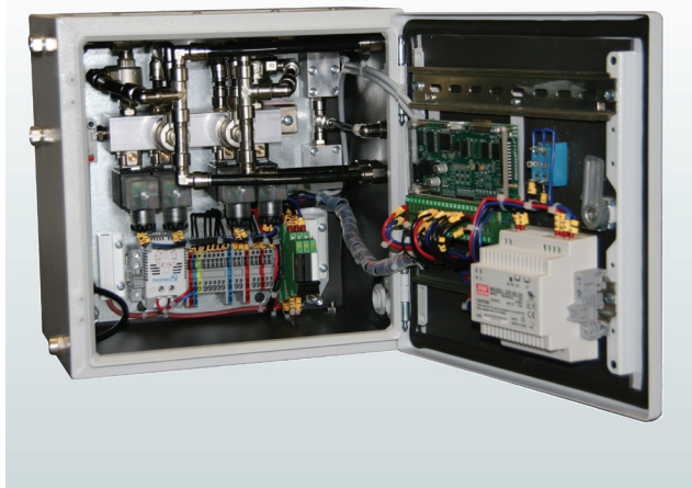
Шкаф управления установкой для запрессовки подшипников Автомобильная промышленность
