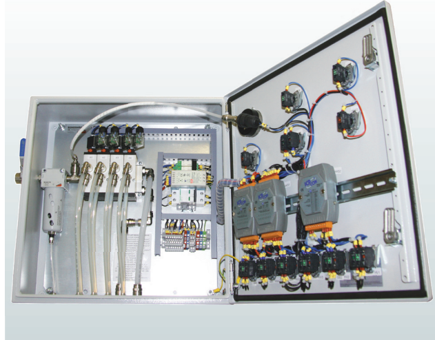
Шкаф управления загрузкой / выгрузкой сыпучих продуктов Строительная отрасль
